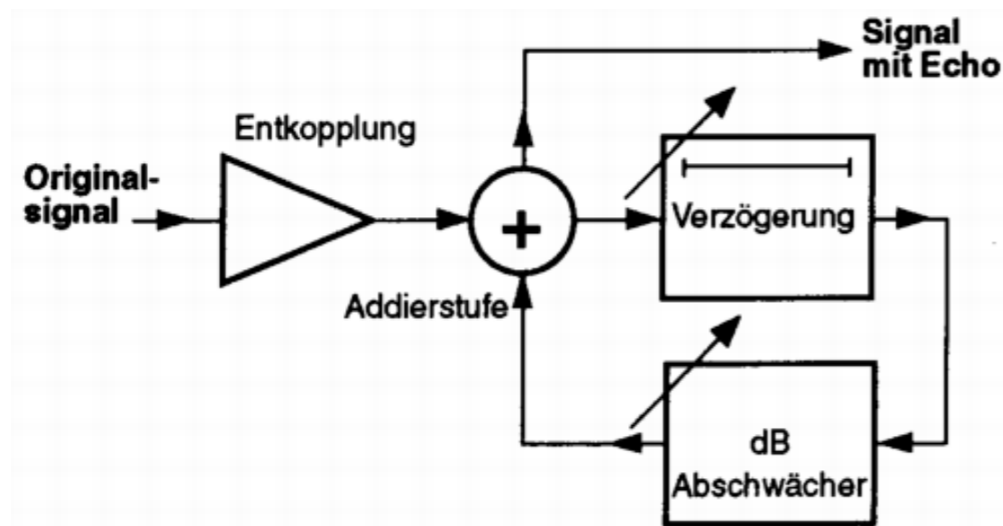
Echoprinzip
