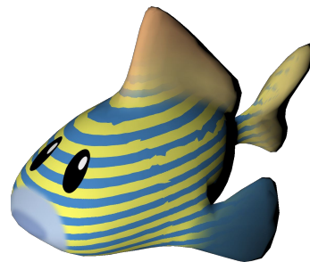
QEM [Garland 1997]
