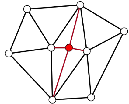
Edge Split
